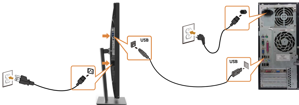
a.连接1台计算机
